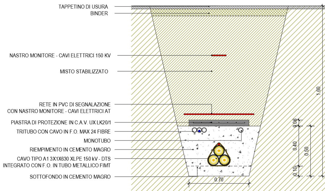
Figura 2 – Sezione tipo scavo in trincea per posa cavidotto 150 kV lungo strada
