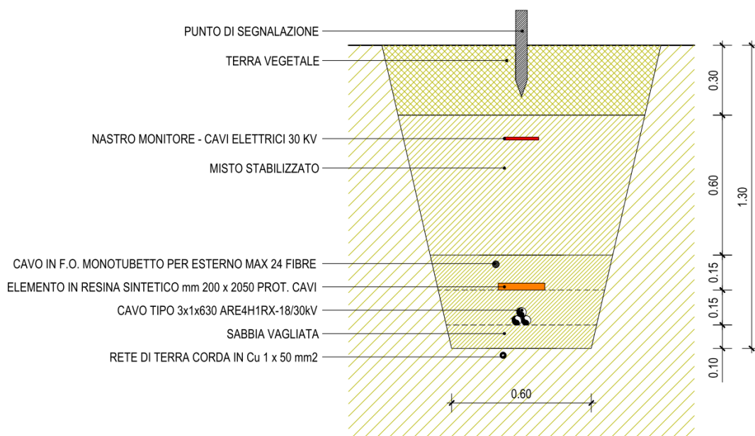
Figura 1 – Sezione tipo scavo in trincea per posa cavidotto 30 kV su terreno agricolo
