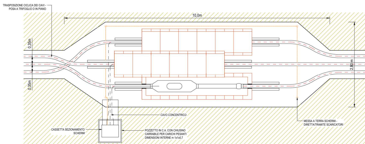
Figura 3 – Schema cameretta giunti
